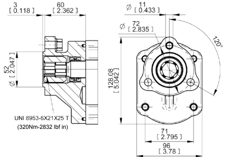
T1 3 BOLT UNI 8953
